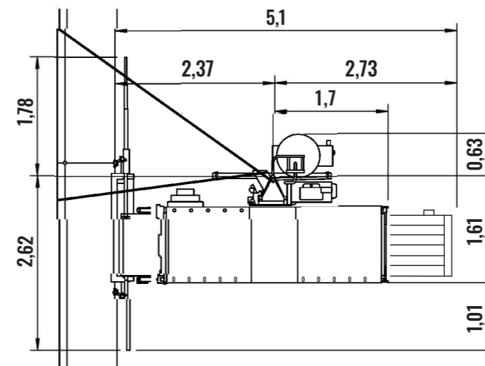
NORMAAL BENODIGDE RUIMTE VOOR STEIGERS
