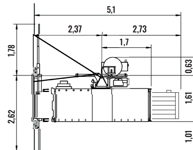
NORMAAL BENODIGDE RUIMTE VOOR MUUR
