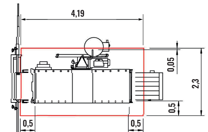
AS-DOORLOPMACHINE (500 MM VANAF RANDEN BINNENPODIUM)
