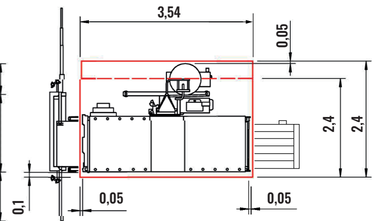
ASMACHINE MET/ZONDER KABELPOT GEEN PERSONENVEROVER
