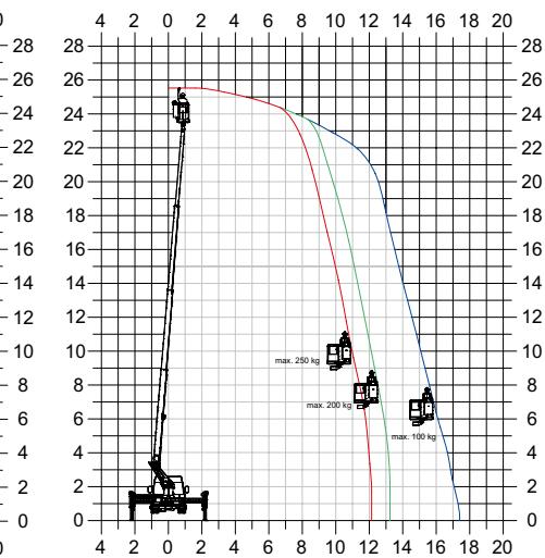
Zijdelingse reikwijdte
